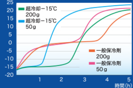
温度(°C) 保冷時間比較試験
